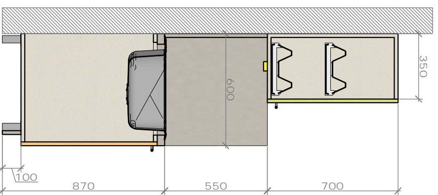
Griezums A-A
