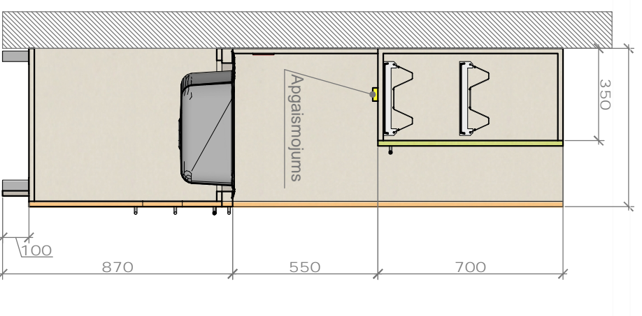
Griezums A-A
