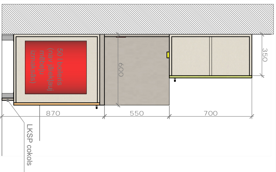
Griezums A-A
