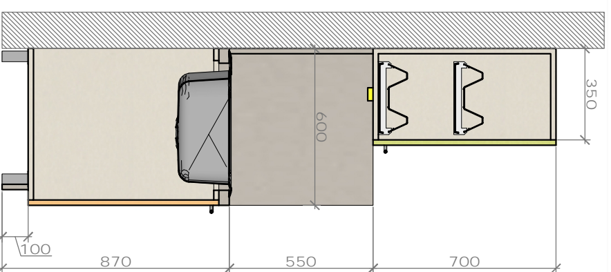
Griezums A-A
